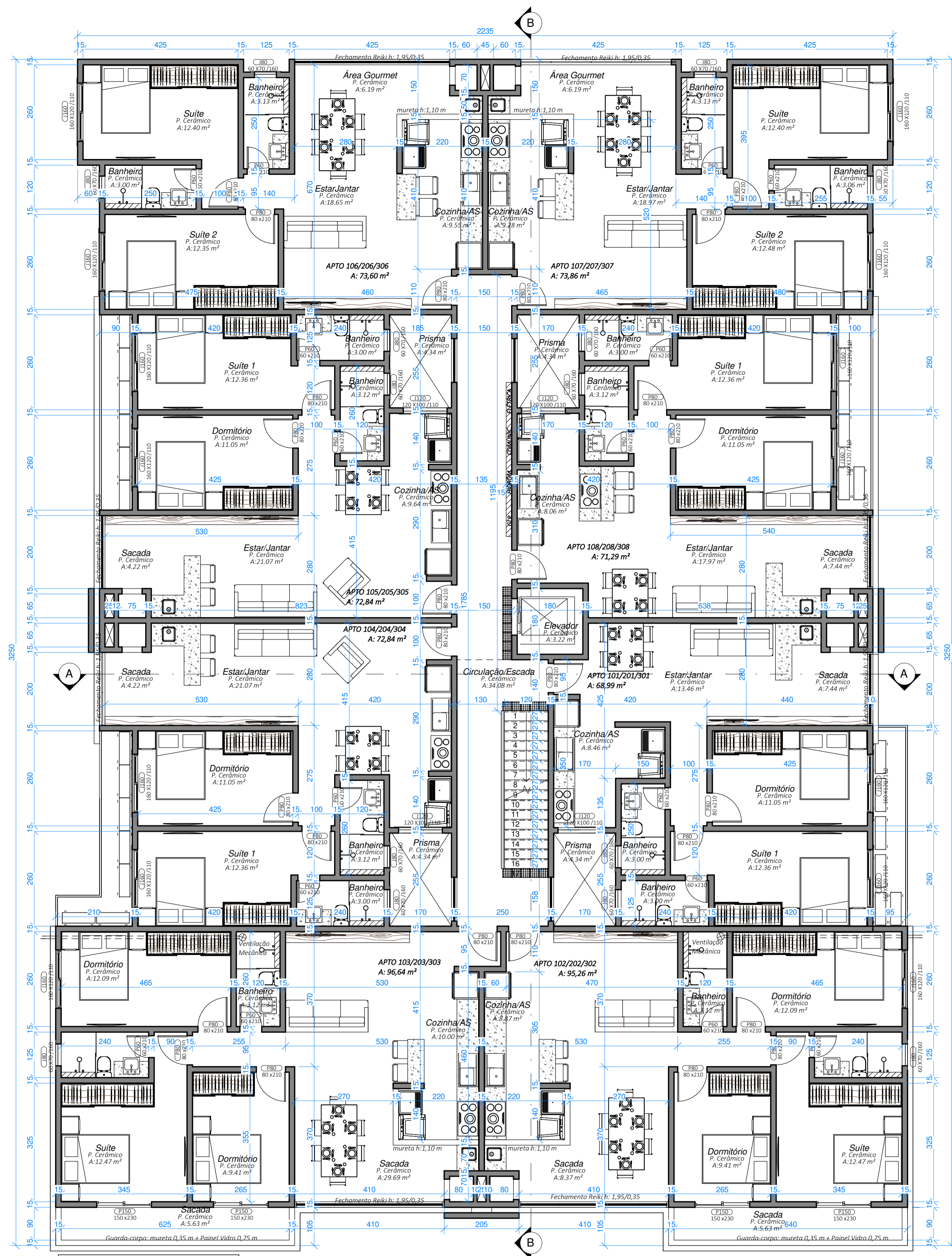
PLANTA BAIXA PAV. PAVIMENTO TIPO X3 A: 667,19 m² ESC 1:75
