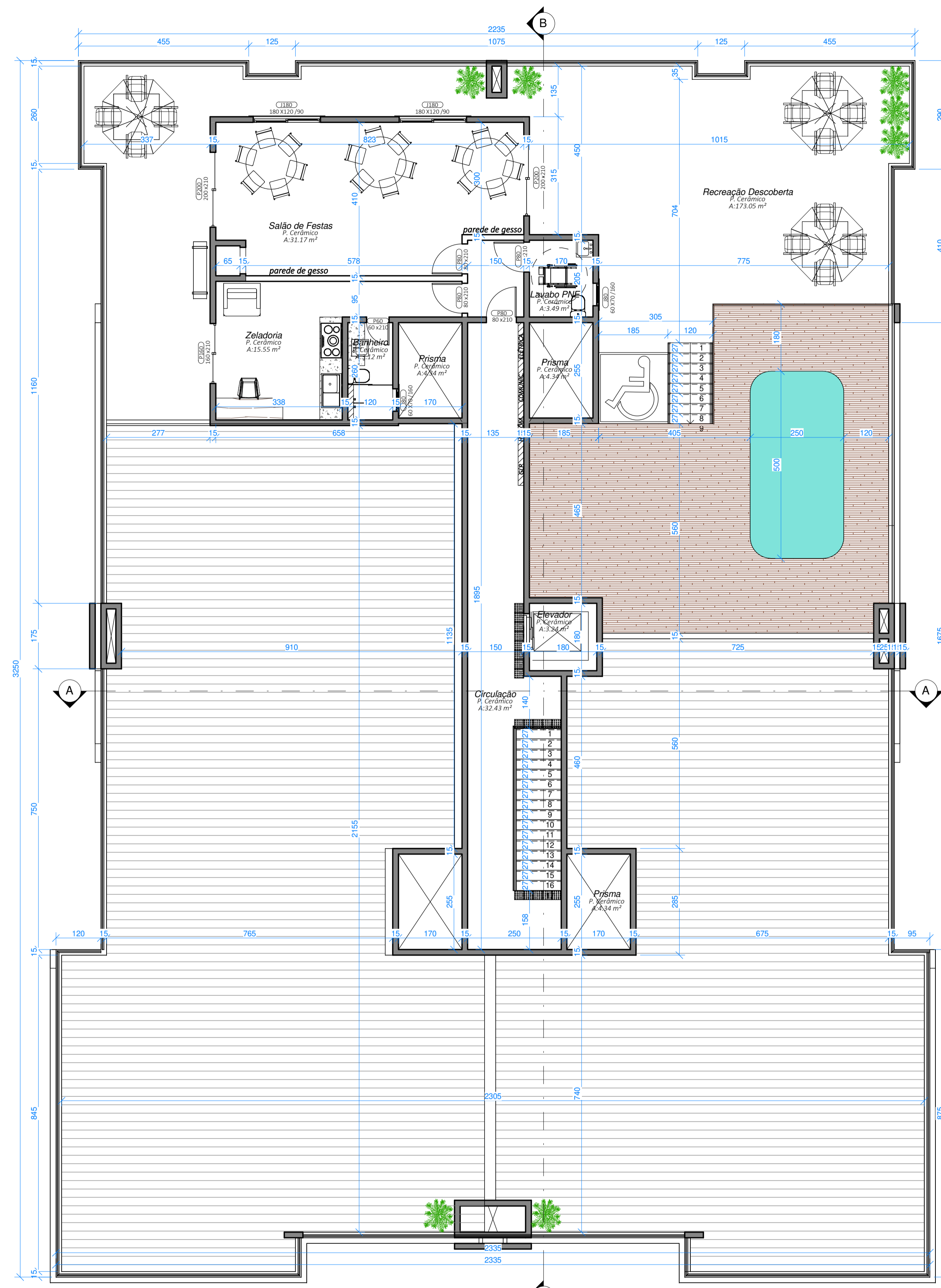
PLANTA BAIXA PAV. PAVIMENTO ÁTICO A: 290,85 m² ESC 1:75
